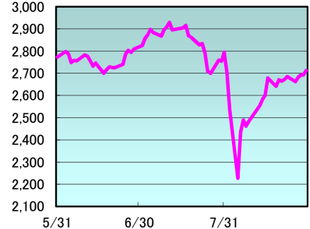
東証株価指数(TOPIX)の3か月の推移
